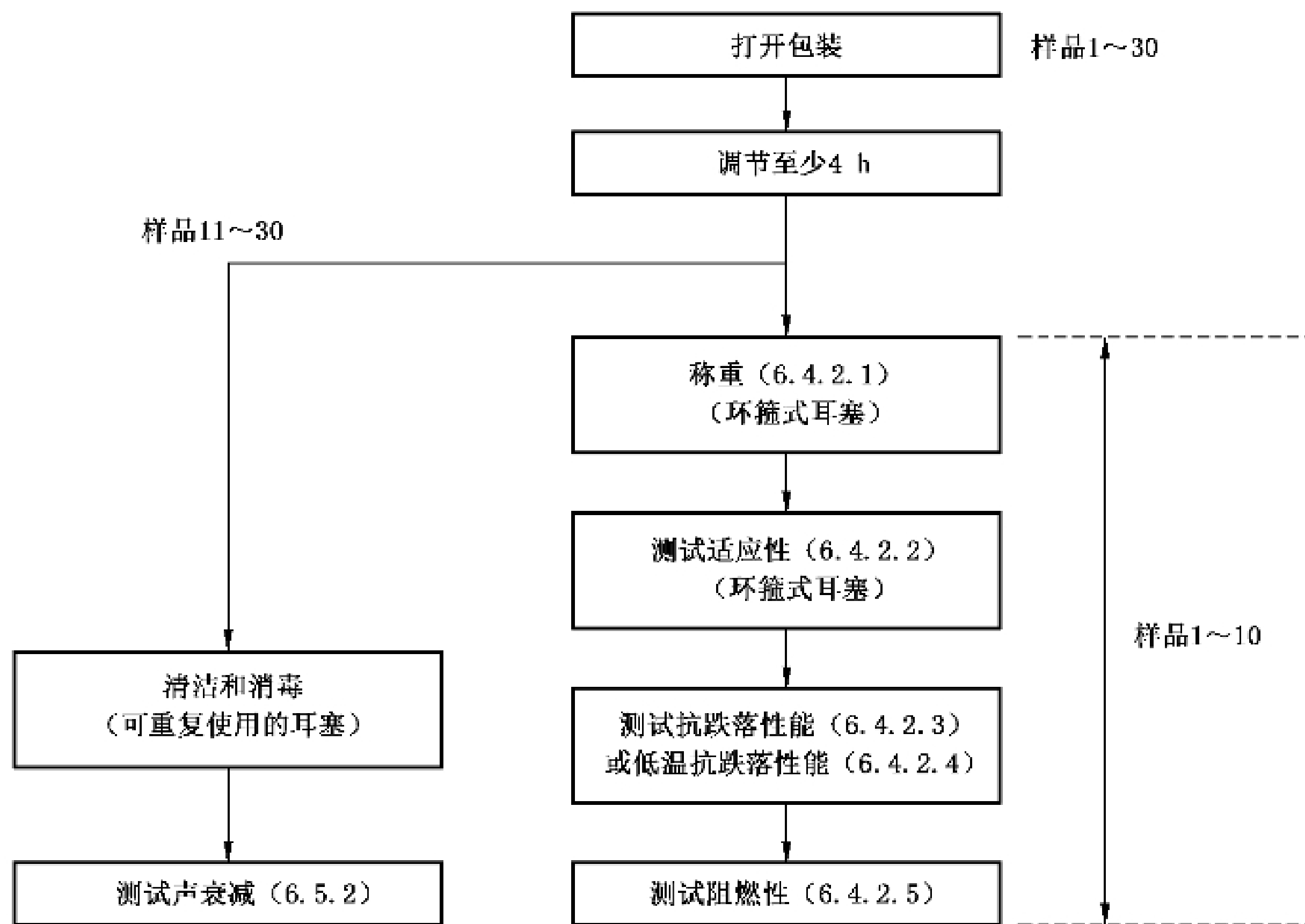
图 B.3 耳塞测试流程图
