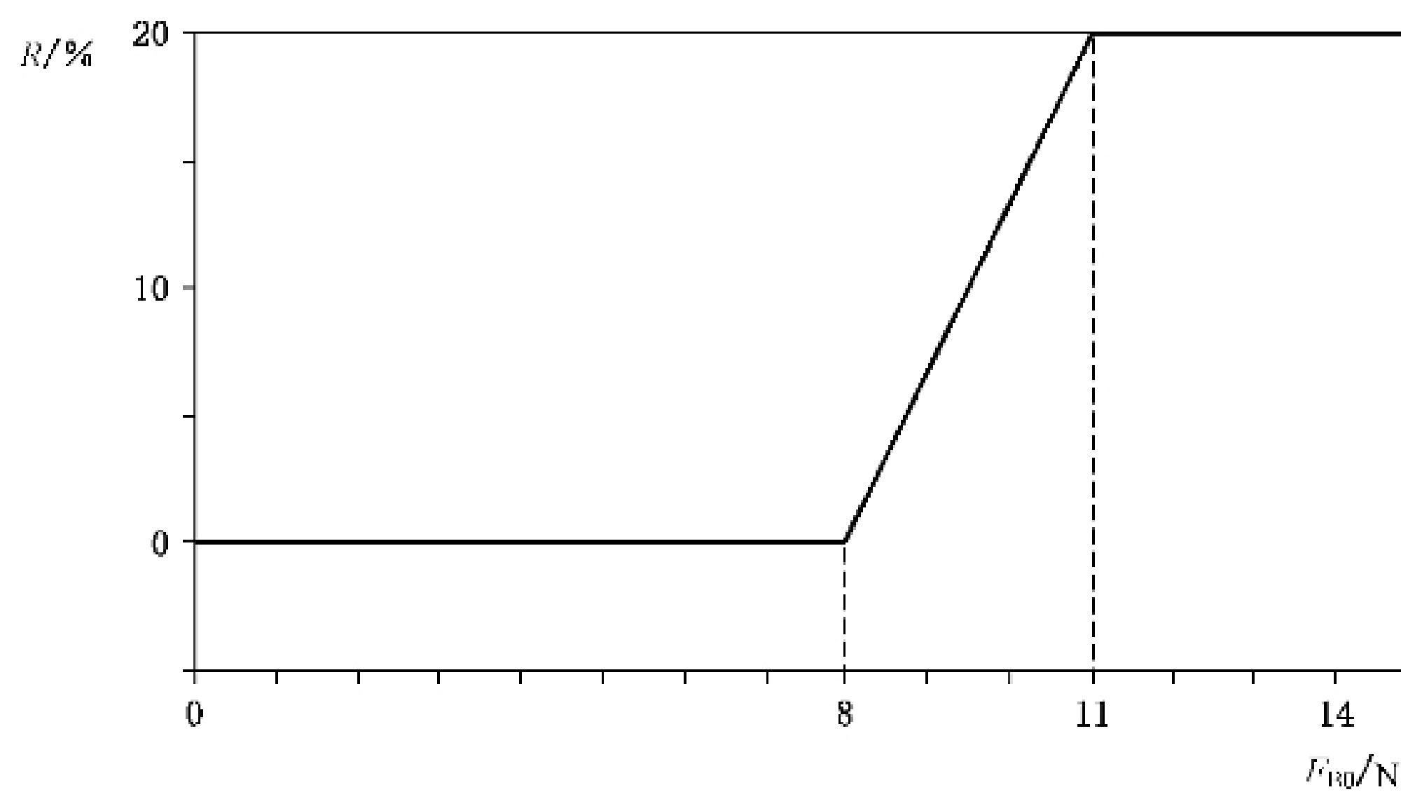
图 10 附加组合夹紧力平均值的最大允许减少百分数
