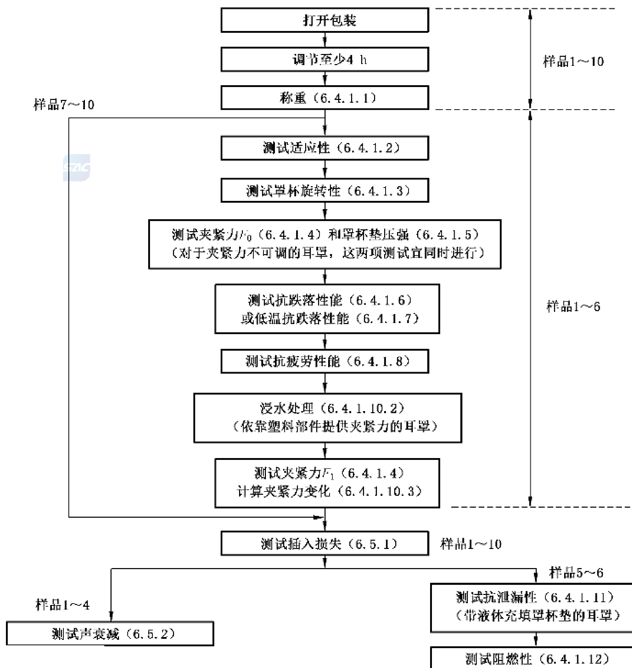
图 B.1 环箍式耳罩测试流程图
